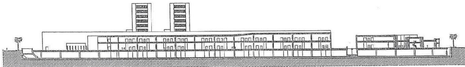
SEZIONE 3-3
