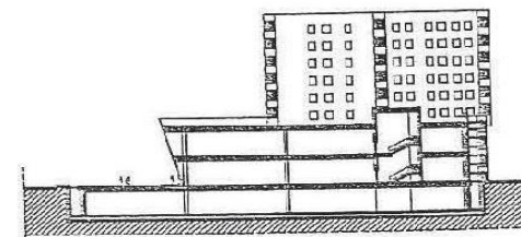
SEZIONE 1-1
