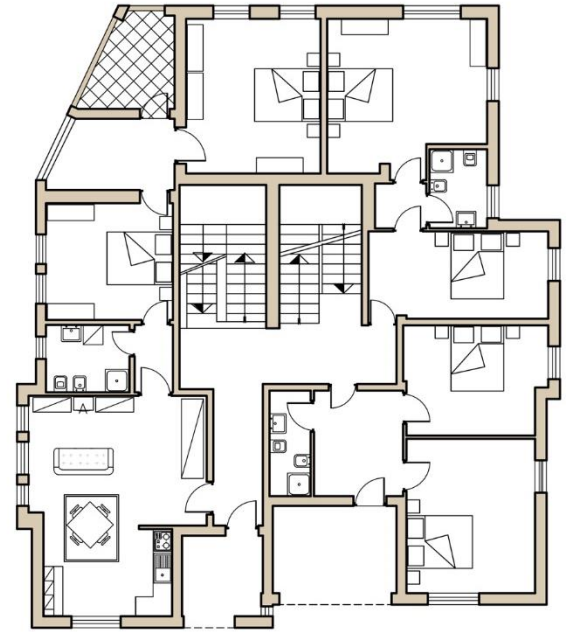
Piano Terra Groundfloor 第一层
