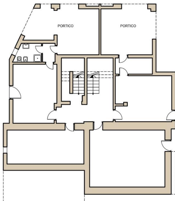
Piano Seminterrato Basement 地下室
